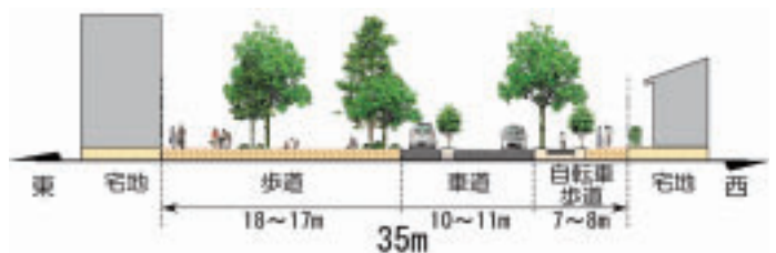
シンボルロードの断面図
