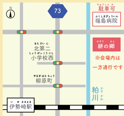
交通案内図
