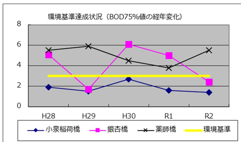
図 3-8 環境基準達成状況 BOD75%値の経年変化 (小泉稻荷橋、銀杏橋、薬師橋)
