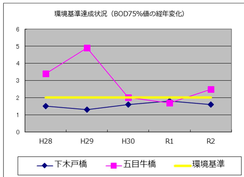
図 3-1 環境基準達成状況 BOD75%値の経年変化（下木戸橋、五目牛橋）
