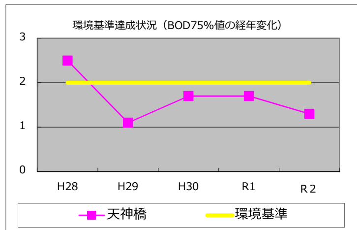
図 3-6 環境基準達成状況 BOD75%値の経年変化（天神橋）
