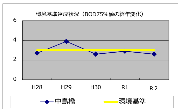
図 3-5 環境基準達成状況 BOD75%値の経年変化 (中島橋)
