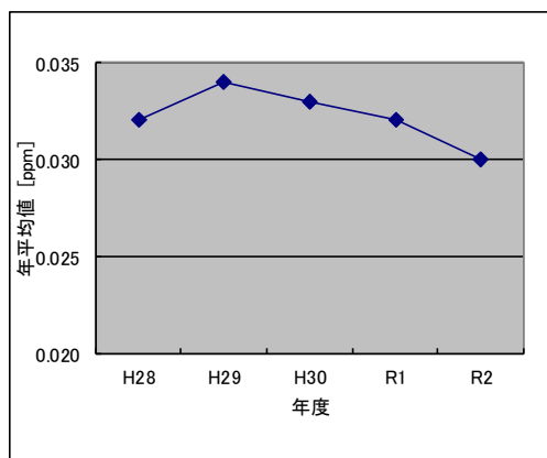
図2-7 光化学オキシダント 経年変化 (昼間1時間値の年平均値)
