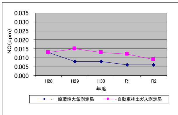
図2-1 一酸化窒素 (NO) 経年変化 日平均値の年間98%値
