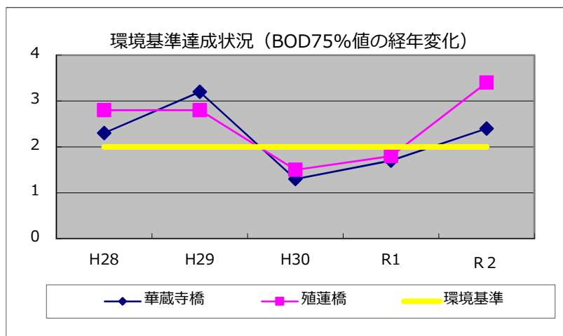
図 3-2 環境基準達成状況 BOD75%値の経年変化（華蔵寺橋、殖蓮橋）
