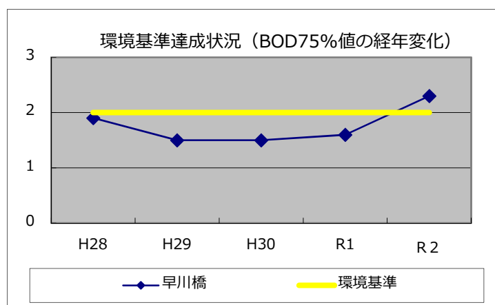
図 3-7 環境基準達成状況 BOD75%値の経年変化 (早川橋)
