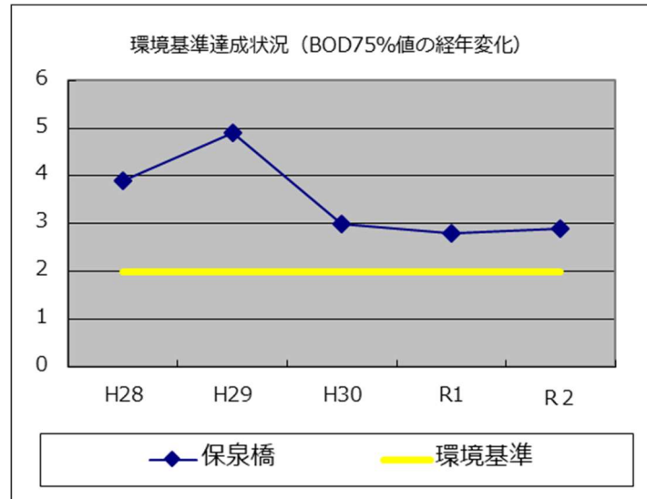
図 3-3 環境基準達成状況 BOD75%値の経年変化 (保泉橋)
