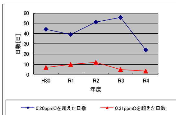
図2-5 非メタン炭化水素 経年変化 (0.20ppmC、0.31ppmCを超えた日数)
