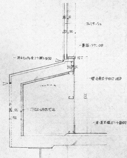
D-13 一般サッシ
