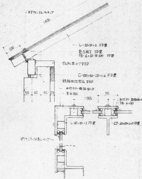
D-29 パラペット S=1:5
