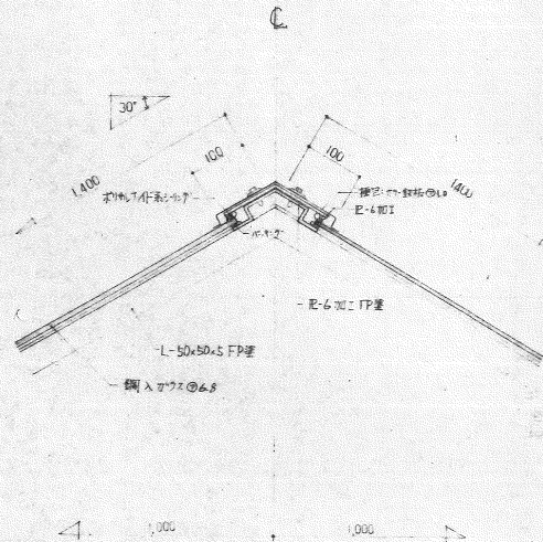
D-26 トーフライト2 S=1:5
