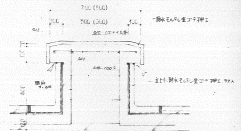
D-32 壁挿被覆詳細(屋内隠取挿のみ) S=1:5
