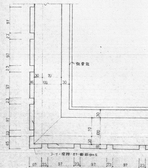
D-15 角波壁 (コーナー)
