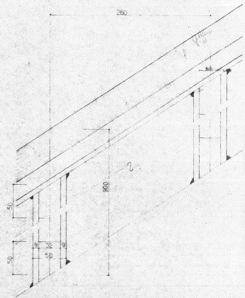
D-14 角波壁 (脚取合)
