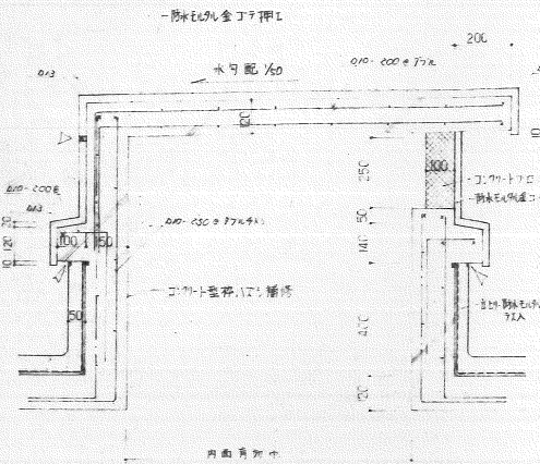
D-31 マラダ上部 S=1:10
