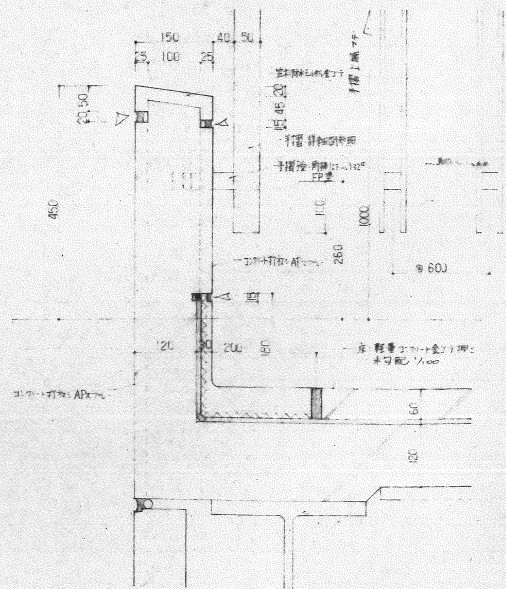
D-30 マラダ S=1:5
