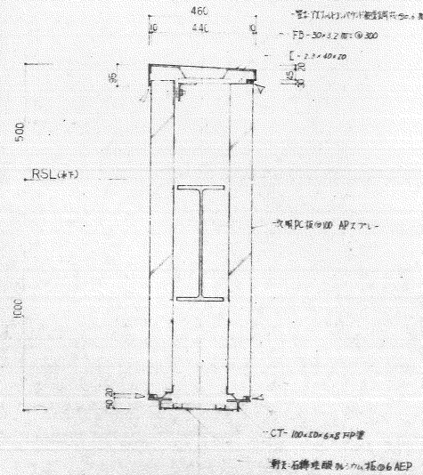
D-31 マラダ上部 S=1:10
