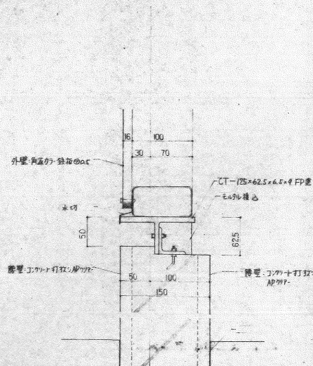
D-14 角波壁 (脚取合)
