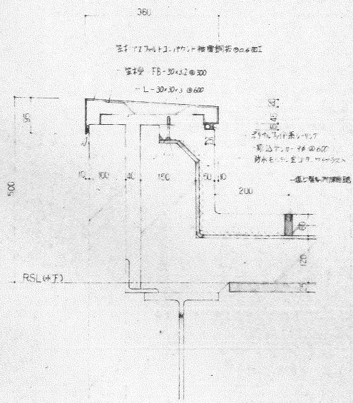
D-29 パラペット S=1:5
