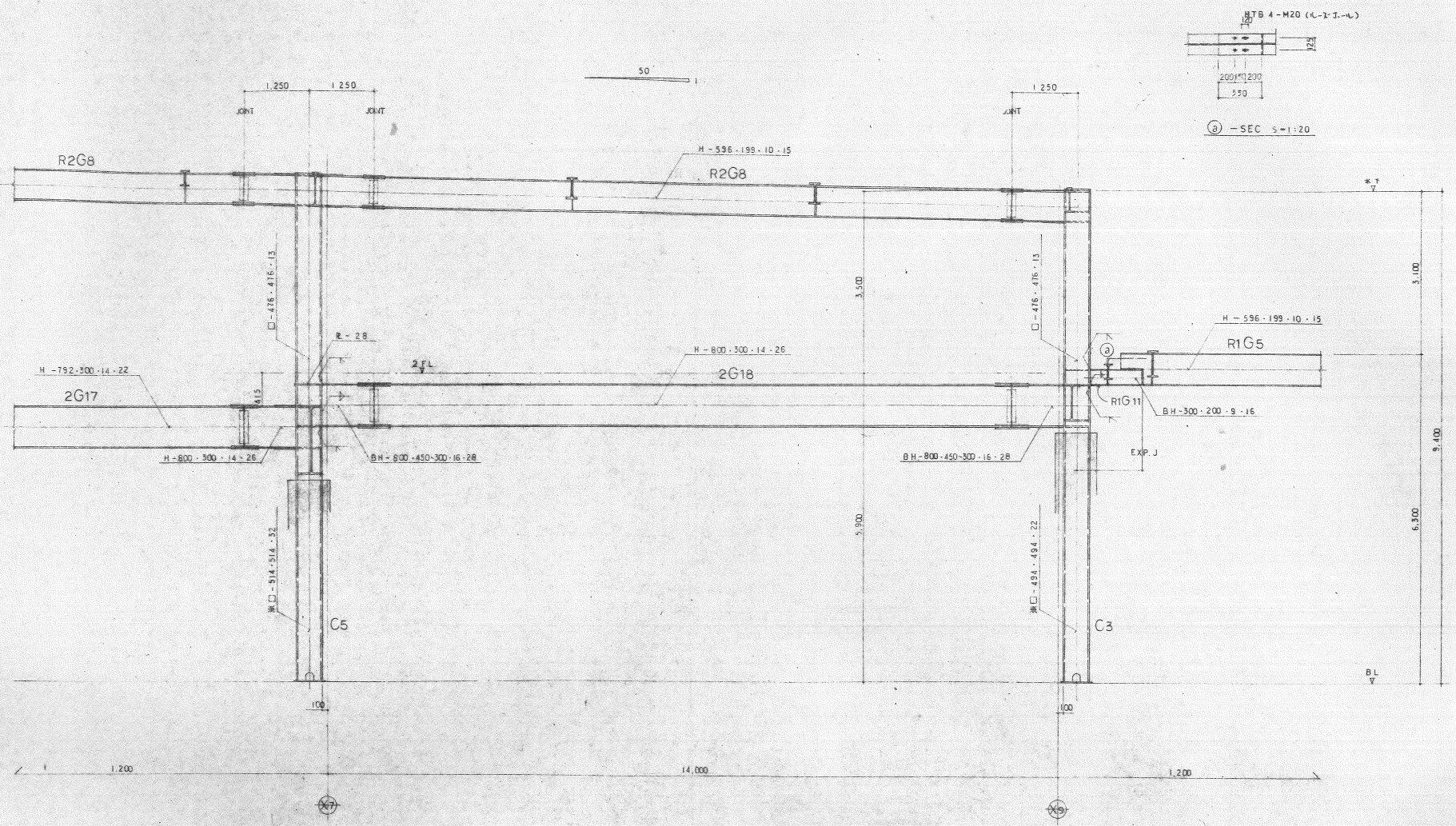
Y4 列柱骨詳圖 S-1:40
