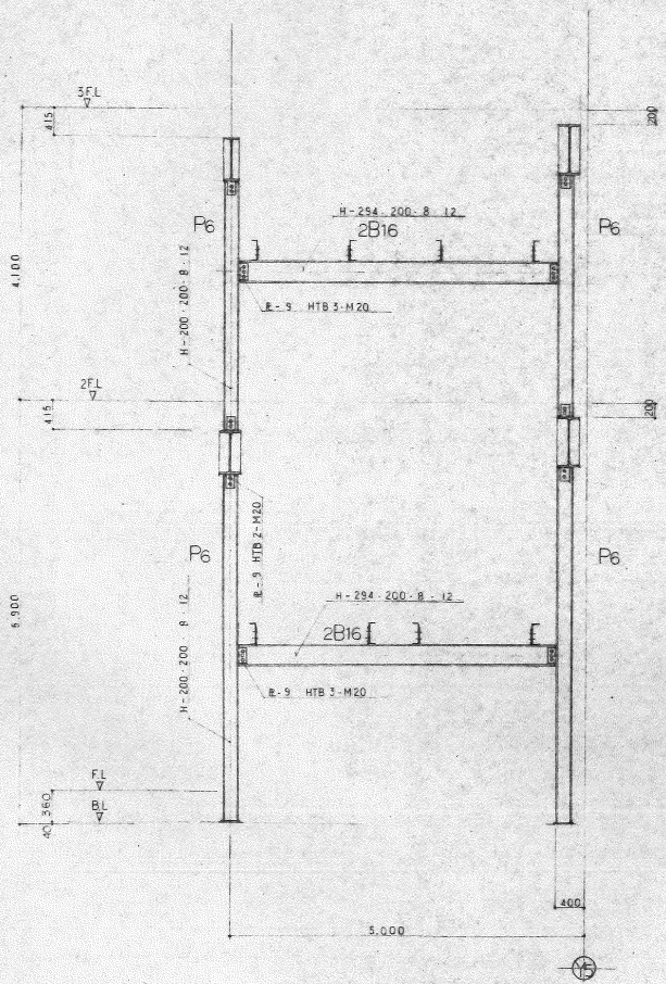
A 階段鉄骨詳細図 S=1:40
