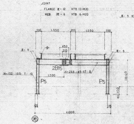
B 鋼梁柱骨節圖 5-1:40
