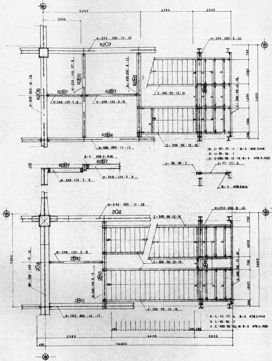
A 階段鉄骨詳細図 9-1:40
