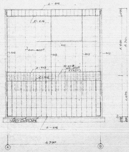
B通りラーメン図 1/30
