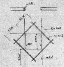
床開口補強 1/30
