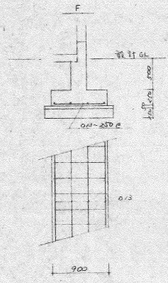
基礎リスト 1/30
