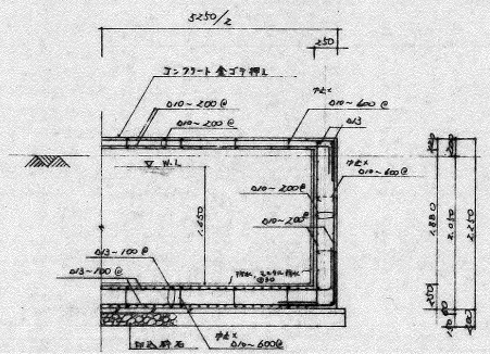
A 断面 1/30
