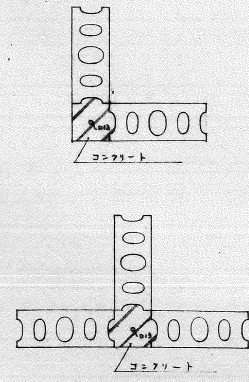
取合詳細図
