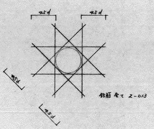
タンポル開口補強
