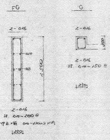
T.V.V配筋詳細図 1/30
