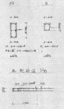
梁リスト 1/30
