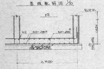
床版配筋図 1/30
