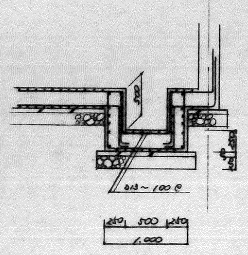
管場配筋図 1/30
