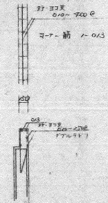
T.V.V配筋詳細図 1/30
