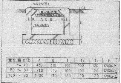
量水器詳細図 NO SCALE
