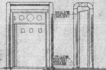
消火栓保護箱詳細図 NO SCALE
