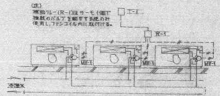
ファンコイル制御(25SETS)
