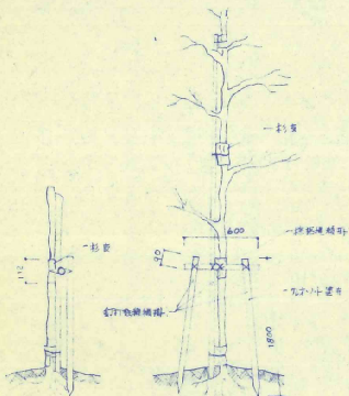
二階型鳥居(赤杉)基礎図
