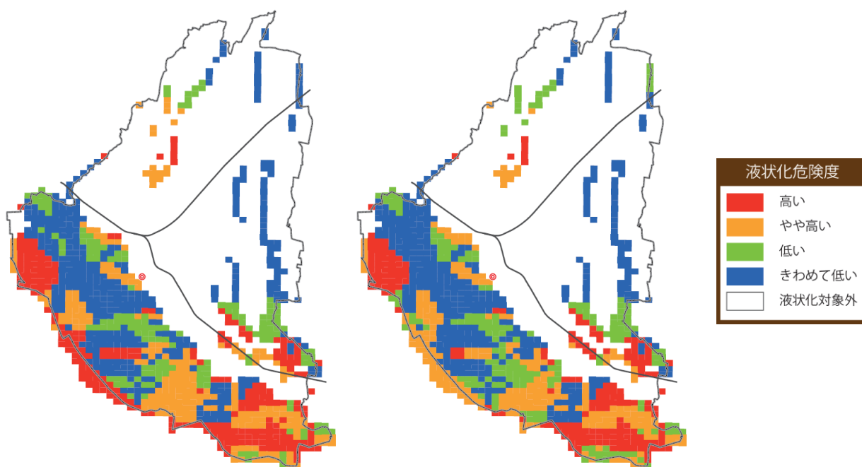
関東平野北西縁断層帯主部 を震源とする地震
