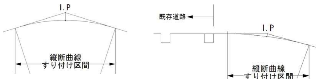
図－13 縦断曲線の設置例
