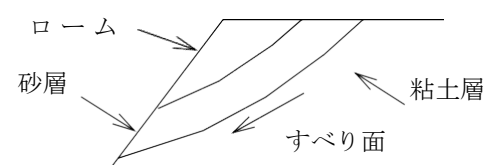
a 層と層とがすべりやすい地盤
