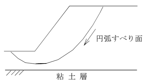
b 円弧すべりが生じやすい地盤
