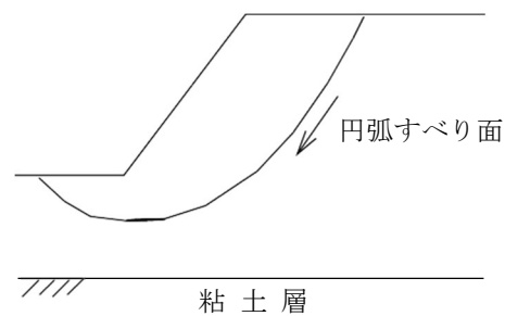
b 円弧すべりが生じやすい地盤
