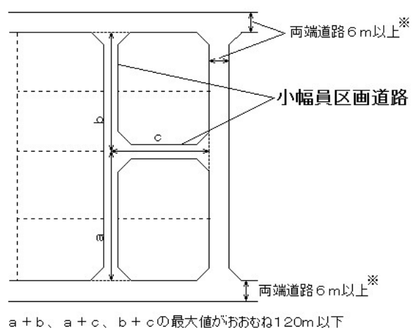
T字状道路の基本形
