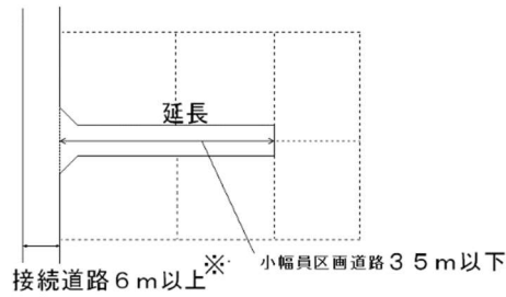
袋路状道路の基本形
