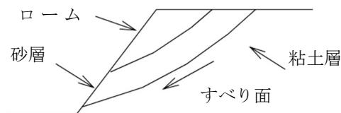
a 層と層とがすべりやすい地盤
