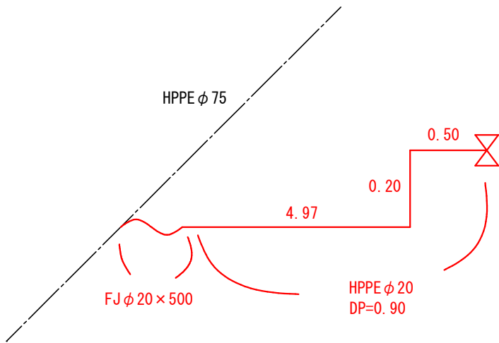
( 立面図 )
