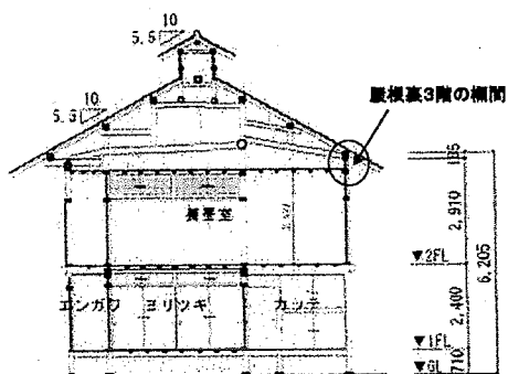
高山家住宅 断面図 (現状断面)
